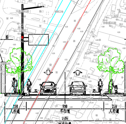
道路标准横断面图 开口道
