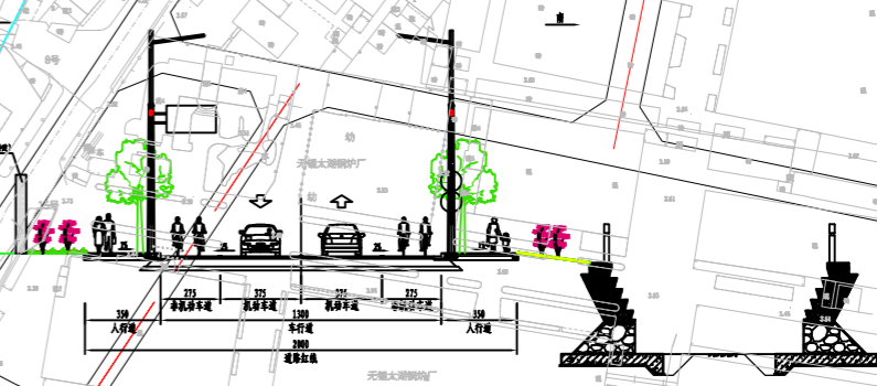
道路标准横断面图 封闭式(非机动车道)
