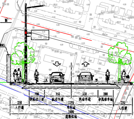
道路标准横断面图 封闭式
